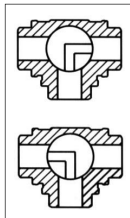
L-Port
